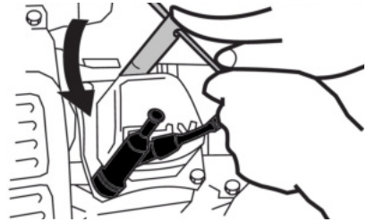
Рис. 21 Обслуживание свечи зажигания
